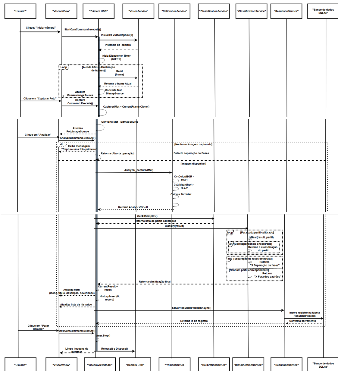
Figura 14 - Diagrama de Sequência Módulo Viscom
