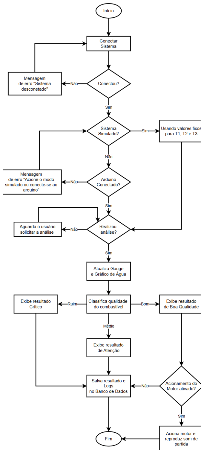
Figura 11 - Diagrama de Fluxo Módulo Tradicional
