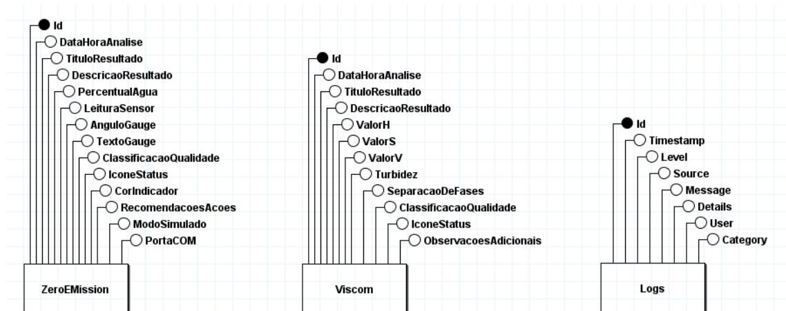
Figura 5 - Modelo Conceitual do Banco de Dados
