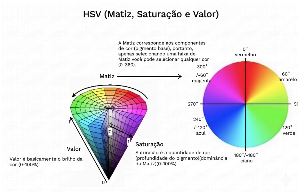
Figura 4 - Modelo HSV
