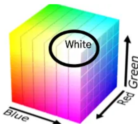
Figura 3 - Modelo RGB
